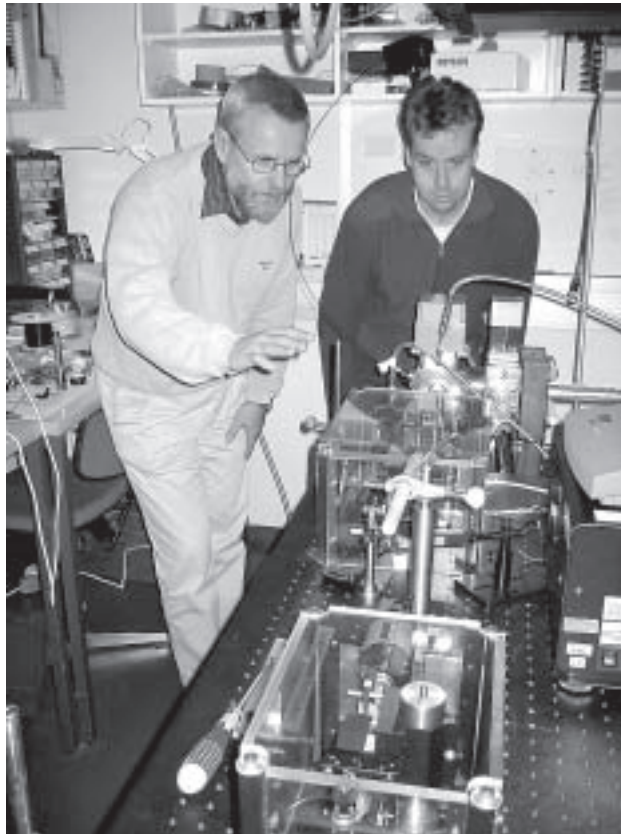
Prof. Rolf Hernberg puuhaamassa laboratoriossa jatko-opiskelija Toni Laurilan rakentaman ulkokaviteettilaserin kanssa.
